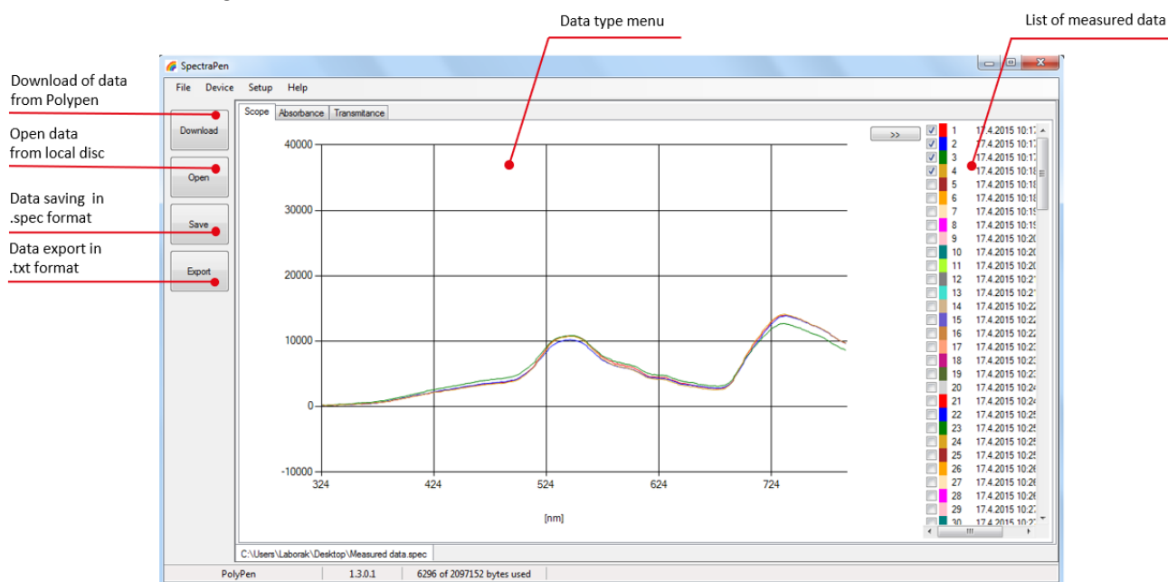
Fig. 27 Scope spectra.
